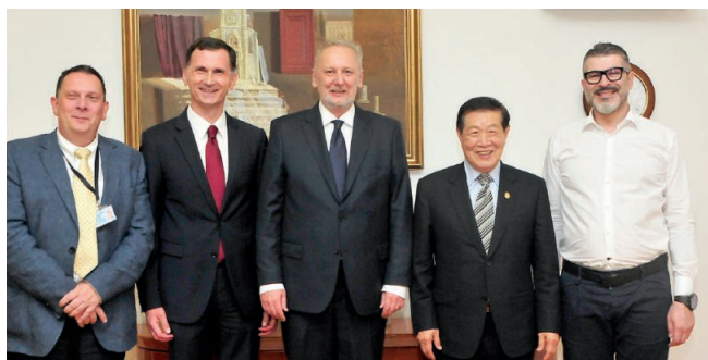
Ministar unutarnjih poslova Davor Božinović i državni tajnik Robert Kopal sastali su se 14. lipnja s proslavljenim svjetskim forenzičarem, dr. Henryjem Chang-Yu Leejem i prof. dr. sc. Draganom Primorcem, jednim od utemeljitelja DNA analize u Hrvatskoj.
